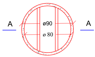
FOSSA SÉPTICA ESCALA - VISUAL
