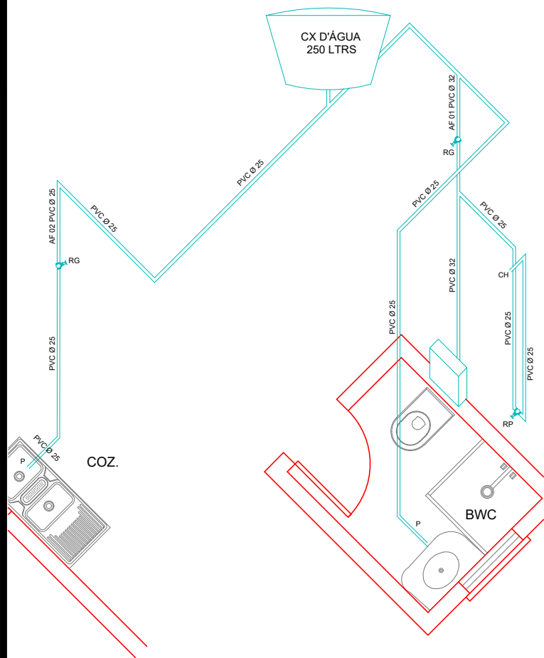
Isométrica Cozinha / Bwc Escala 1/50
