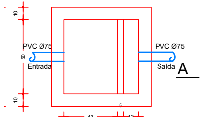
PLANTA BAIXA CAIXA DE GORDURA ESCALA.....S/N
