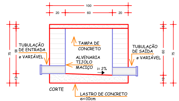
CAIXA DE INSPEÇÃO ESCALA.....S/N
