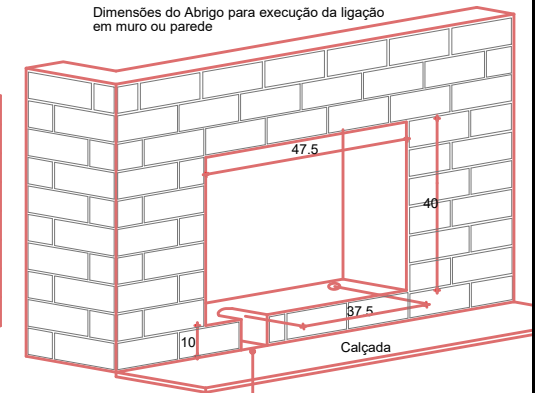
Detalhes do Abrigo para instalação do Cavalete para ligação d'Água Escala Não Indicada
