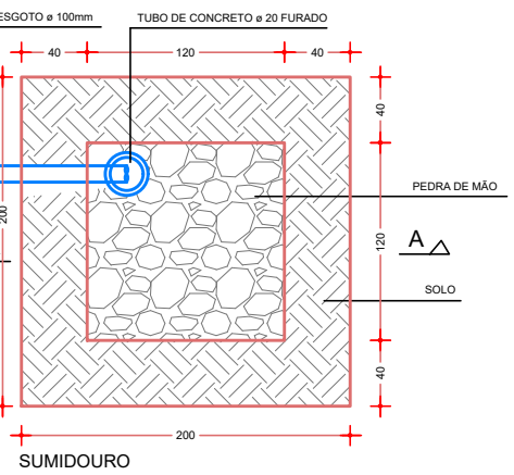
PLANTA BAIXA SUMIDOURO ESCALA - VISUAL
