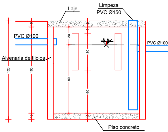
FOSSA SÉPTICA CORTE AA ESCALA - VISUAL
