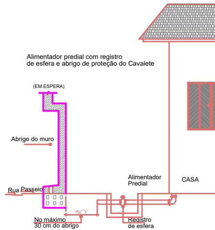
Detalhes do Abrigo para instalação do Cavalete para ligação d'Água Escala Não Indicada
