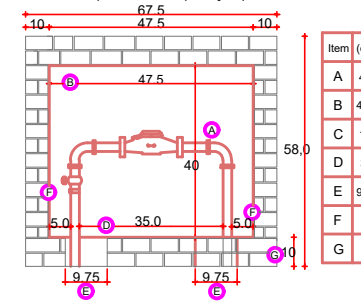
Detalhes do Abrigo para instalação do Cavalete para ligação d'Água Escala Não Indicada
