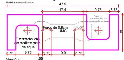
Gabarito da Base do Abrigo - Para instalação do Cavalete.
