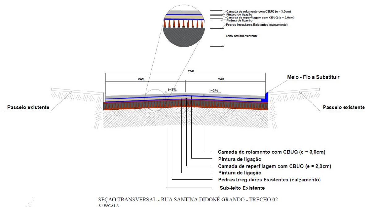
Detalhe 02 – Execução de pavimentação sobre calçamento
