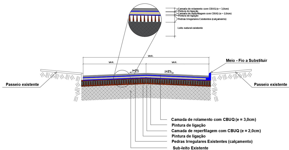
SEÇÃO TRANSVERSAL - RUA SANTINA DIDONÉ GRANDO - TRECHO 01 S / ESCALA
