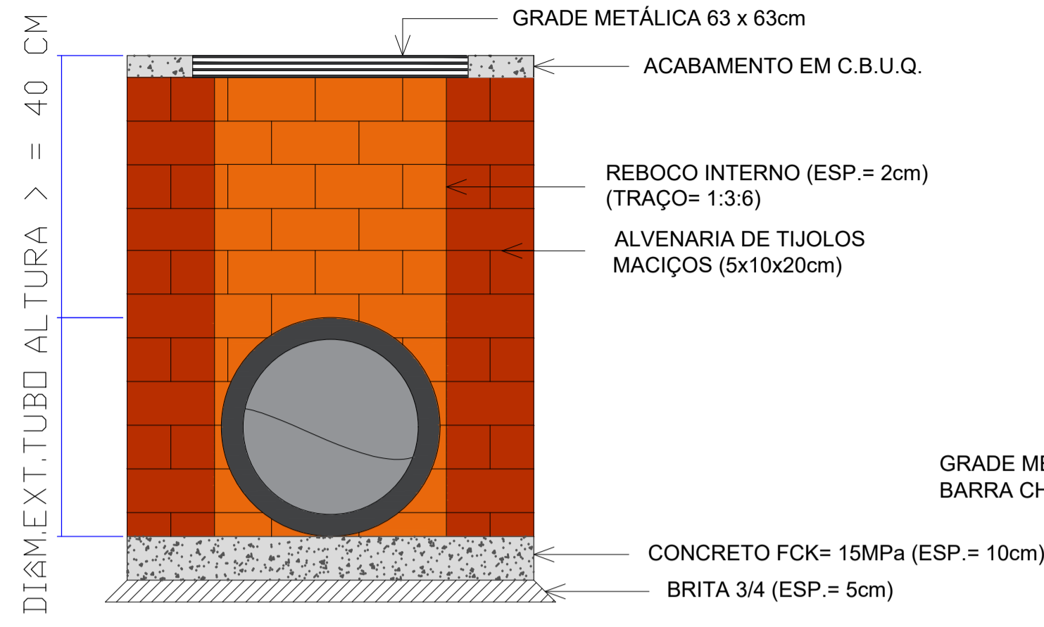
CORTE A-A
