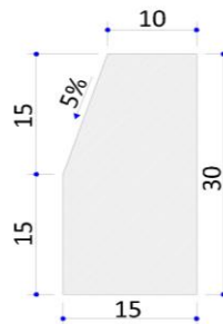
Detalhe 02 – Meio Fio Simples Extrusado
