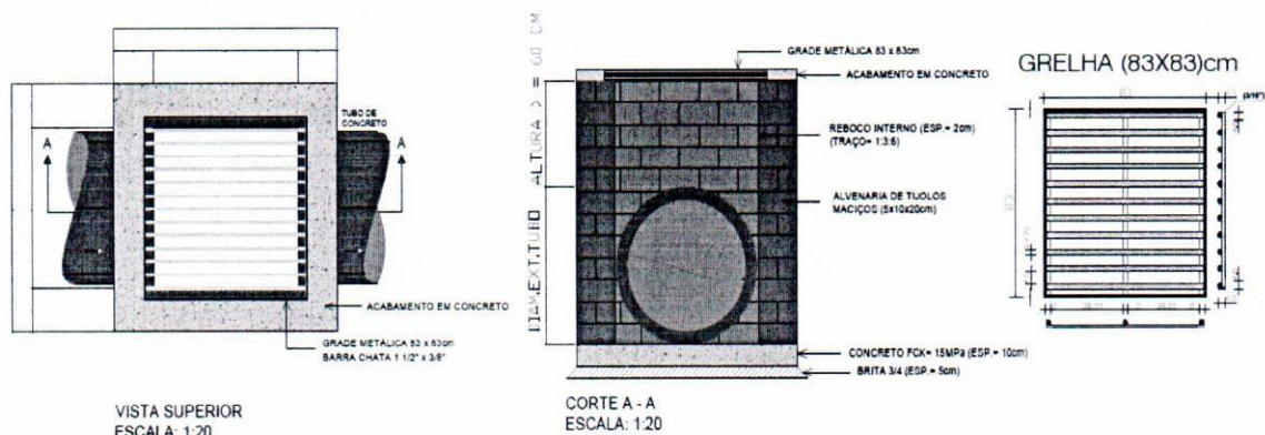
Detalhe 02 – Detalhe Boca de Lobo Ø60cm
