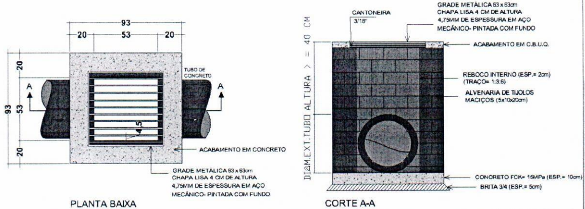
Detalhe 01 – Detalhe Boca de Lobo Ø40cm
