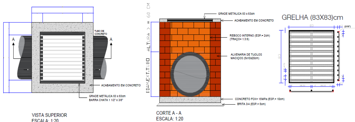
Detalhe 02 – Detalhe Boca de Lobo Ø60cm
