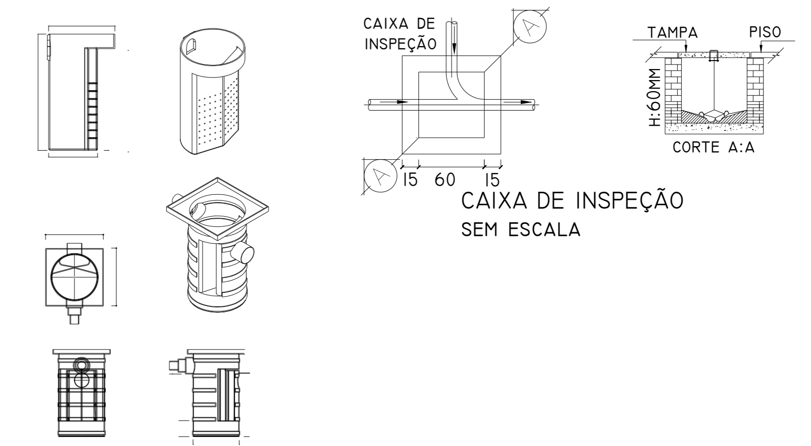
CAIXA DE GORDURA - 120L
