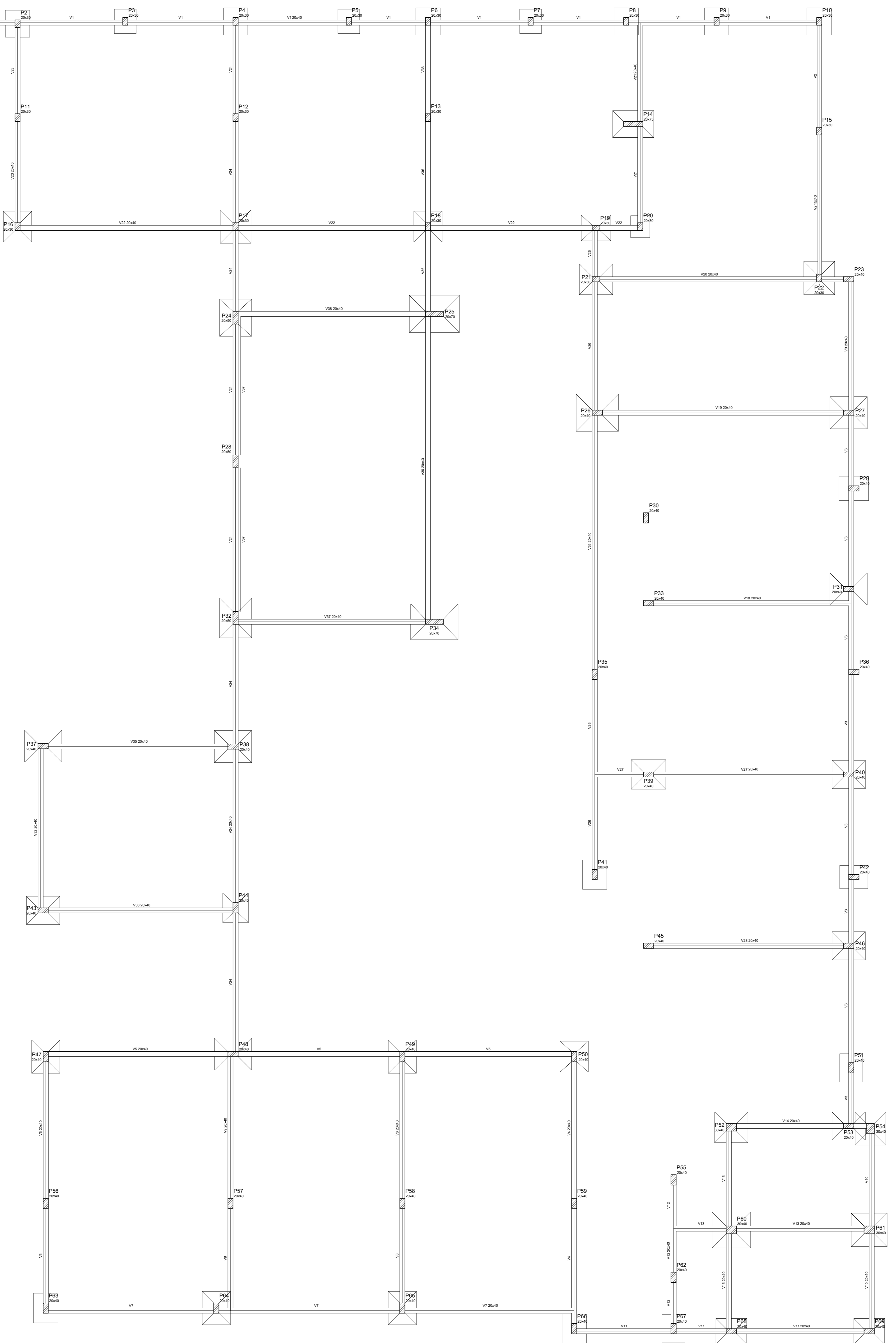
Forma do pavimento BALDRAME escala 1:50
