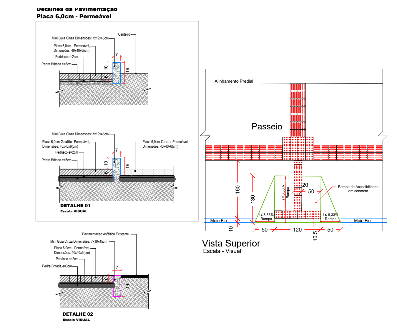
Modelo de pavimentação a ser executado * A mesma deve ser com juntas desencontradas
