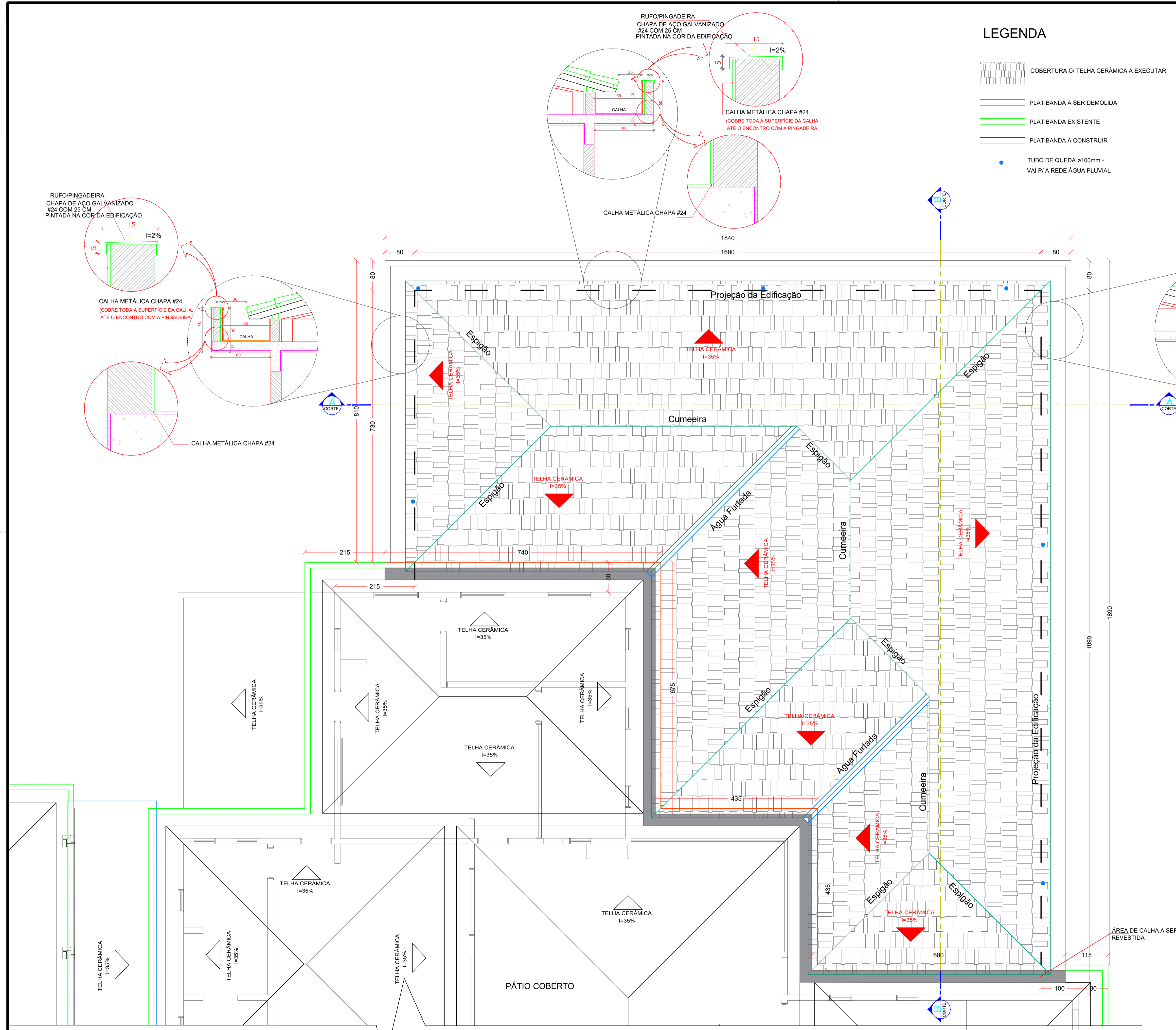
Planta de Cobertura Escala 1/50
