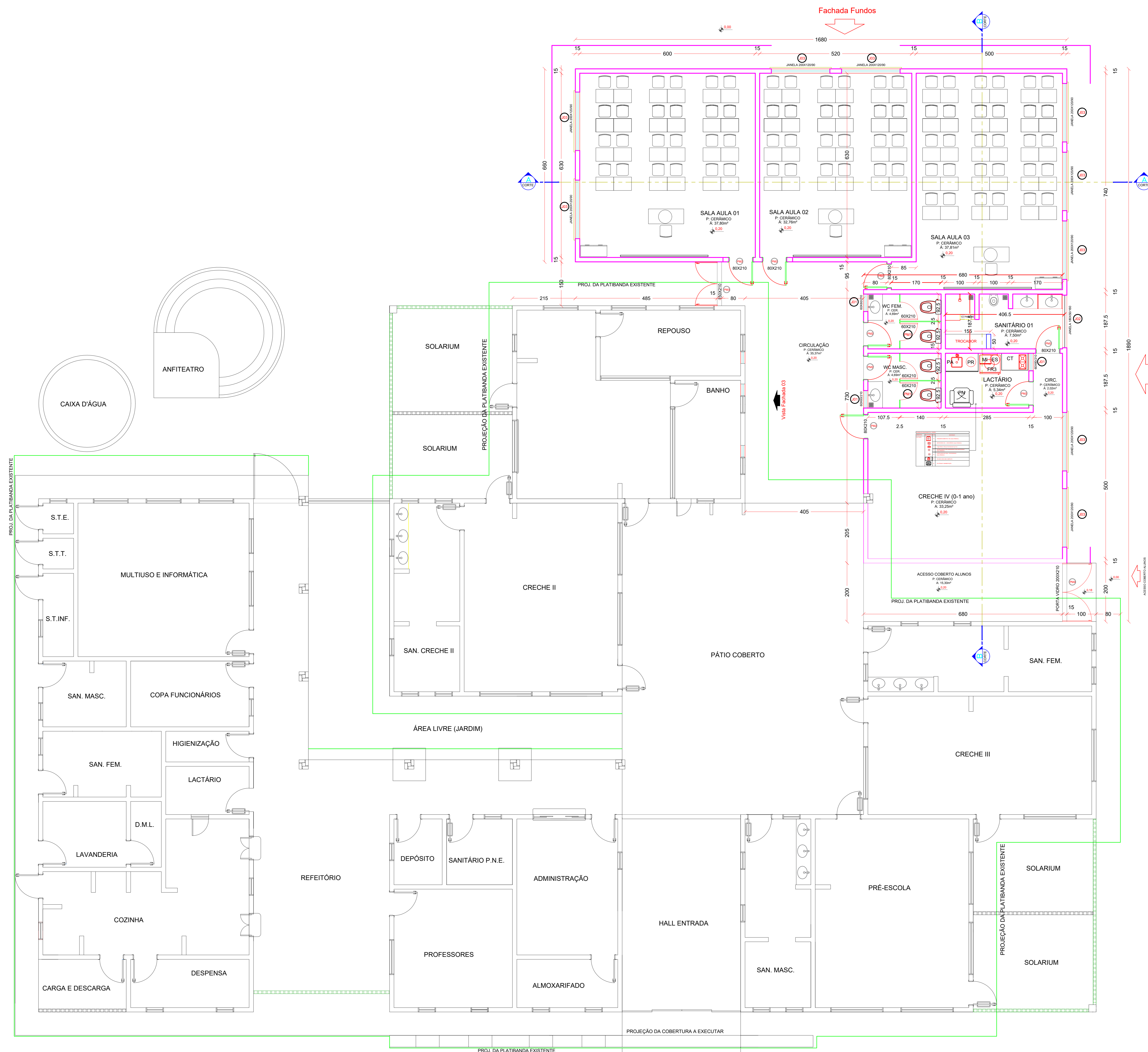
Planta Baixa Escala 1/50 Área a Ampliar = 231,20m²
