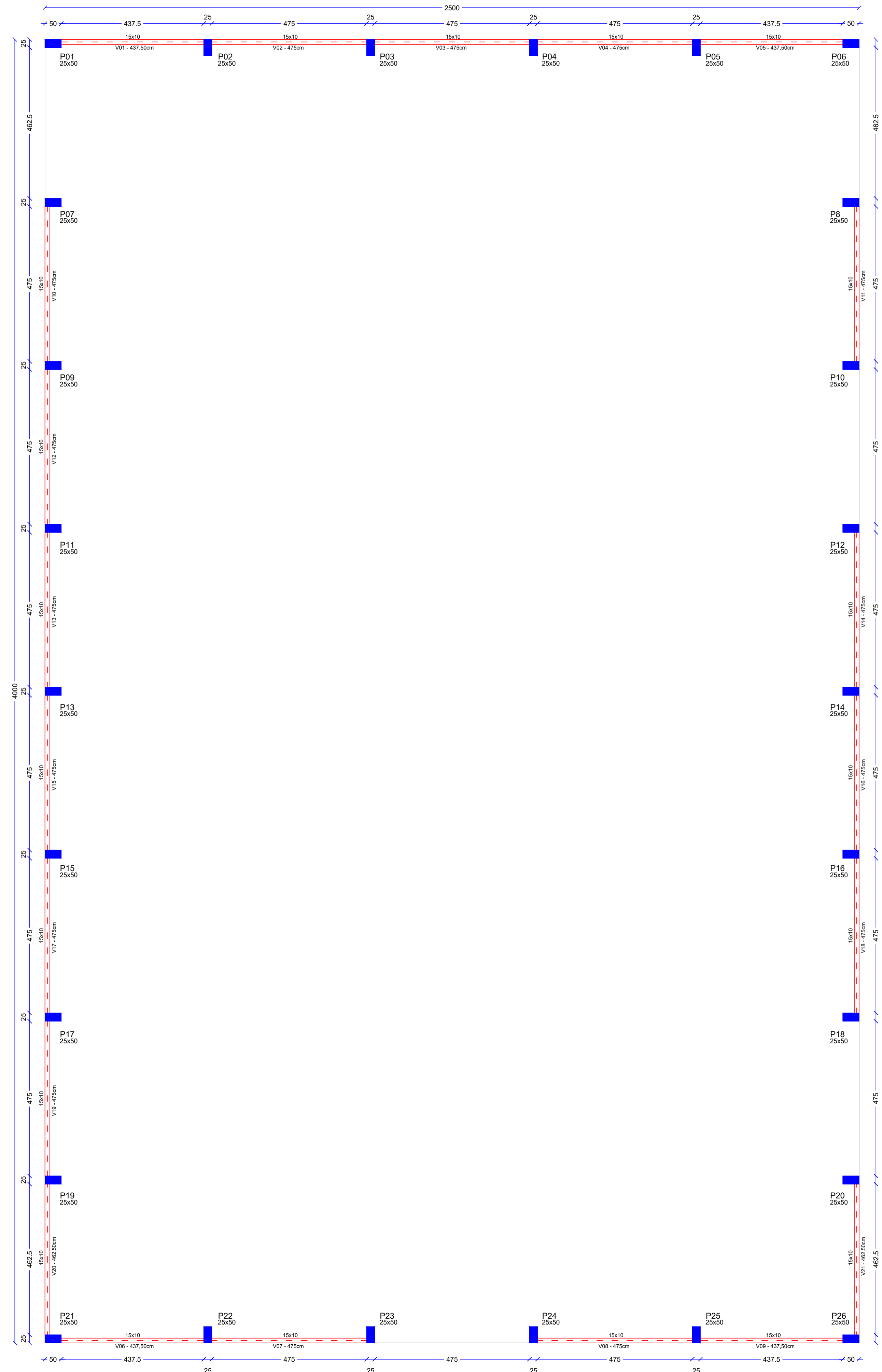
Planta de Vigas Intermediarias (Moldadas "In Loco")
